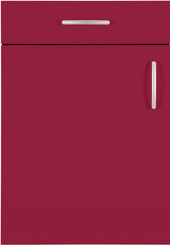
Front: F 208 Burgundrot Frontmaterial: 16 mm Dekorspanplatte Kante: 4-seitig 2 mm ABS, dekorgleich
